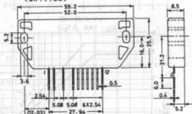
外形図 4055 (unit:mm)
